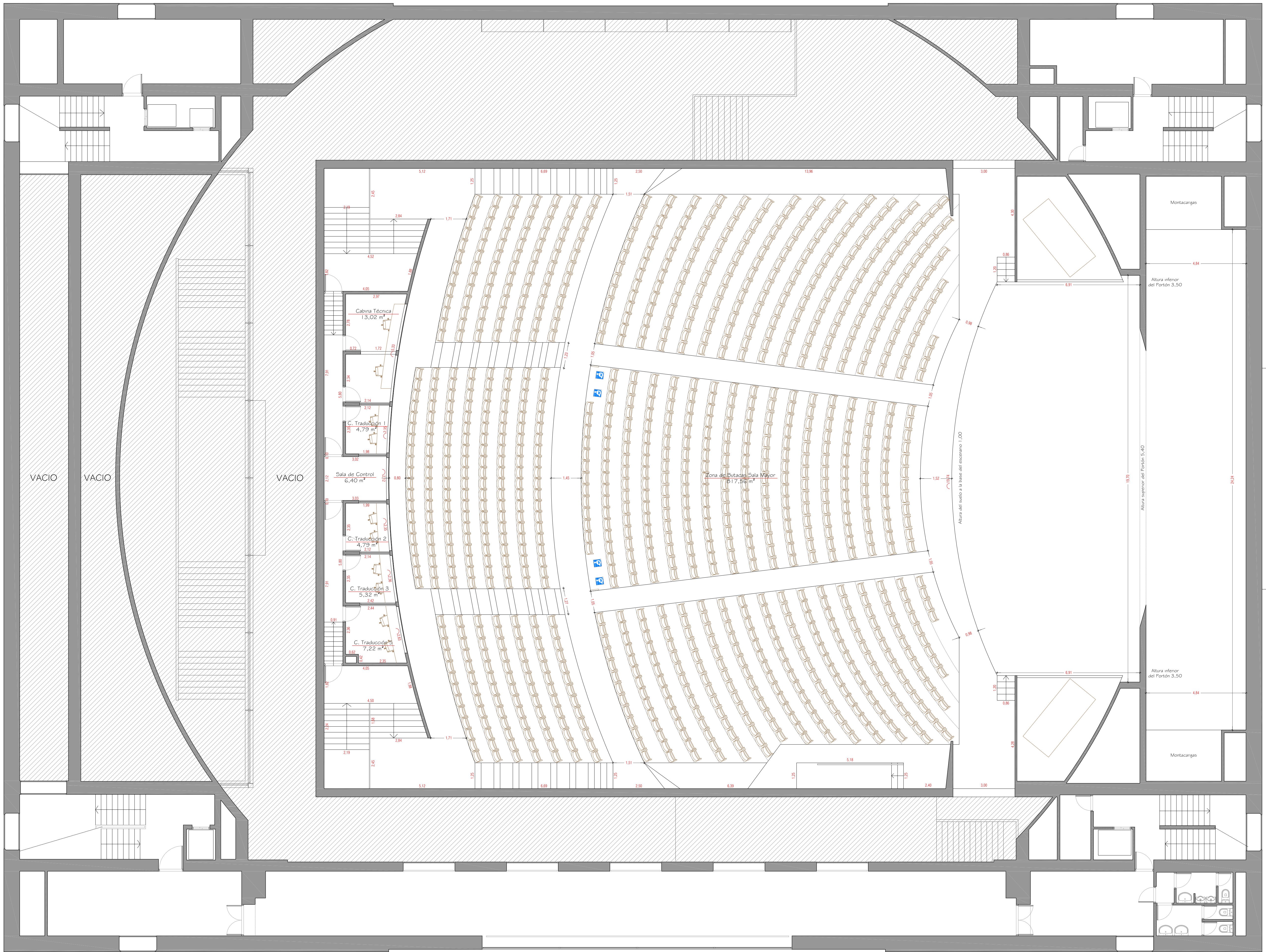
PLANTA NIVEL 4, COTA +3,30 Y +3,50
